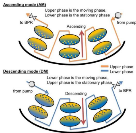
Abbildung 1: Schema einer CPC im aufsteigenden bzw. absteigenden Modus (Örkényi 2017).
